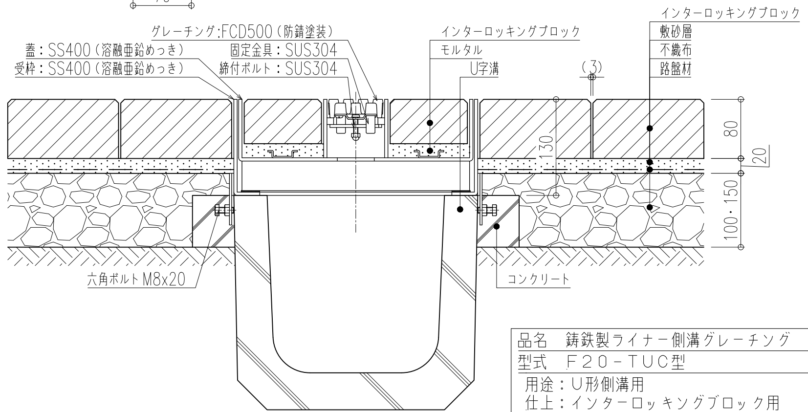
施工参考図
